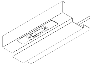
REV. FLUSH BOLT PREP.
